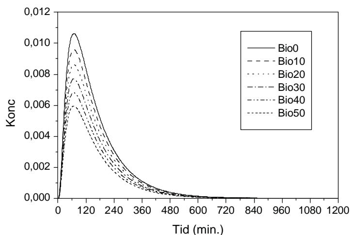
Konc. i vandløb ved forskellig rensningsprocent i biofilter
